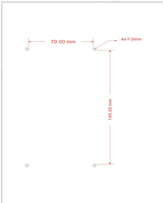
FY100 门禁机防水罩一孔位安装图
